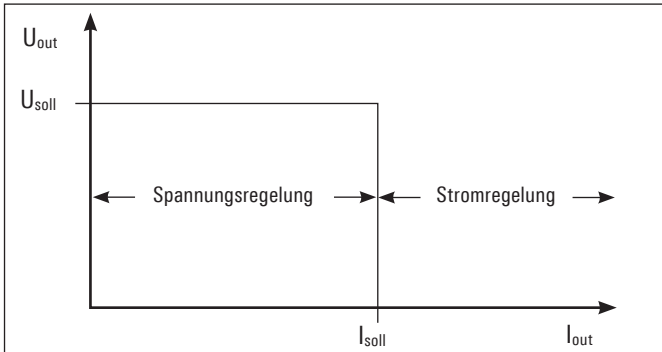
Abb. 4.5: Strombegrenzung
